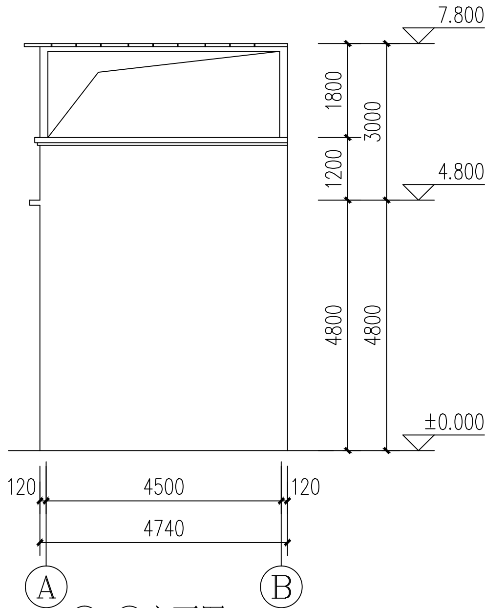
①-②立面图 1:100
