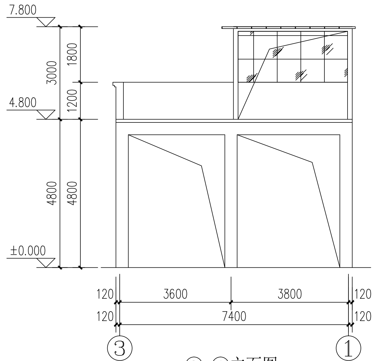
③-①立面图 1:100
