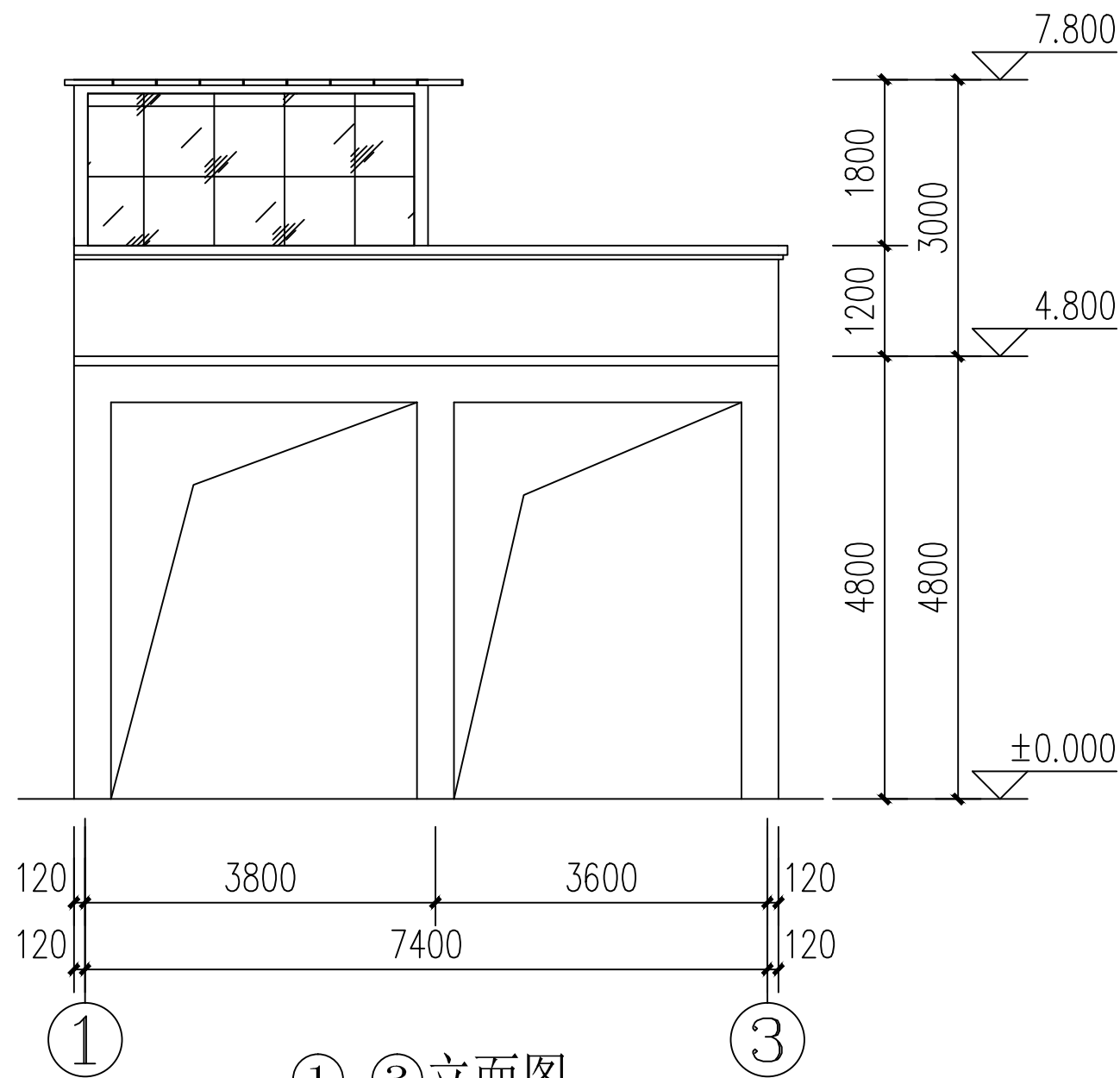
①-③立面图 1:100
