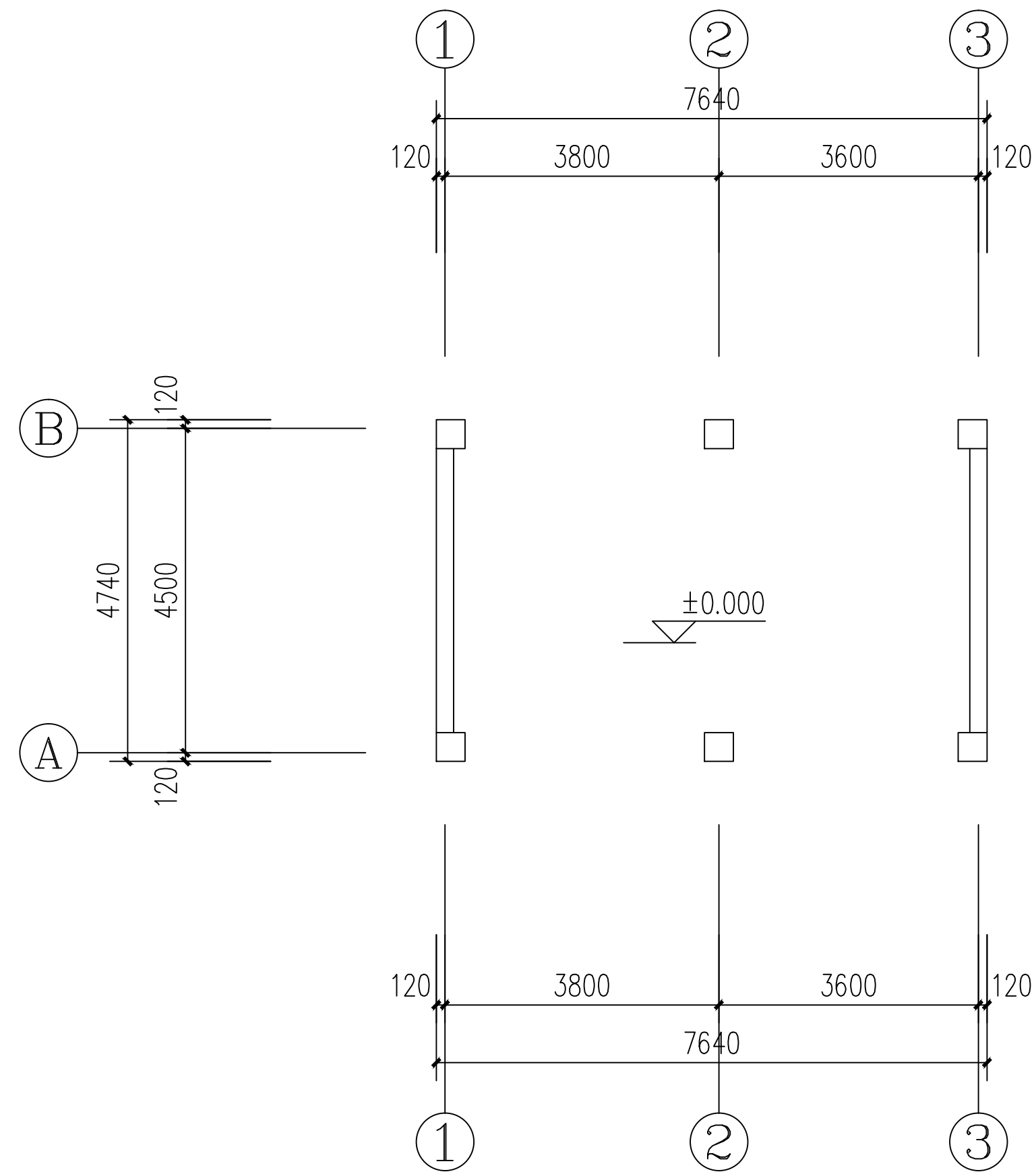
一层平面图 1:100
