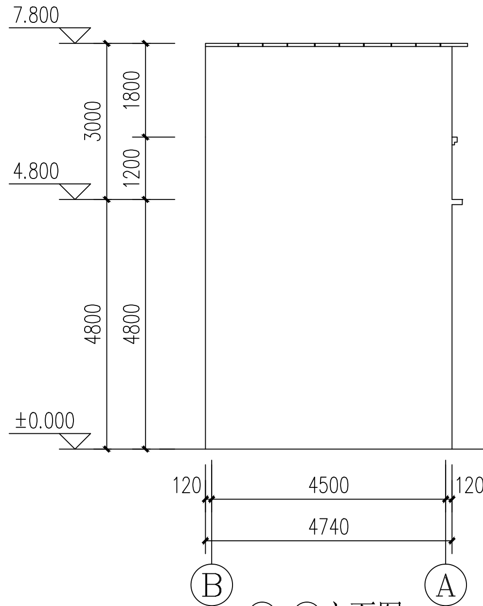
②-①立面图 1:100
