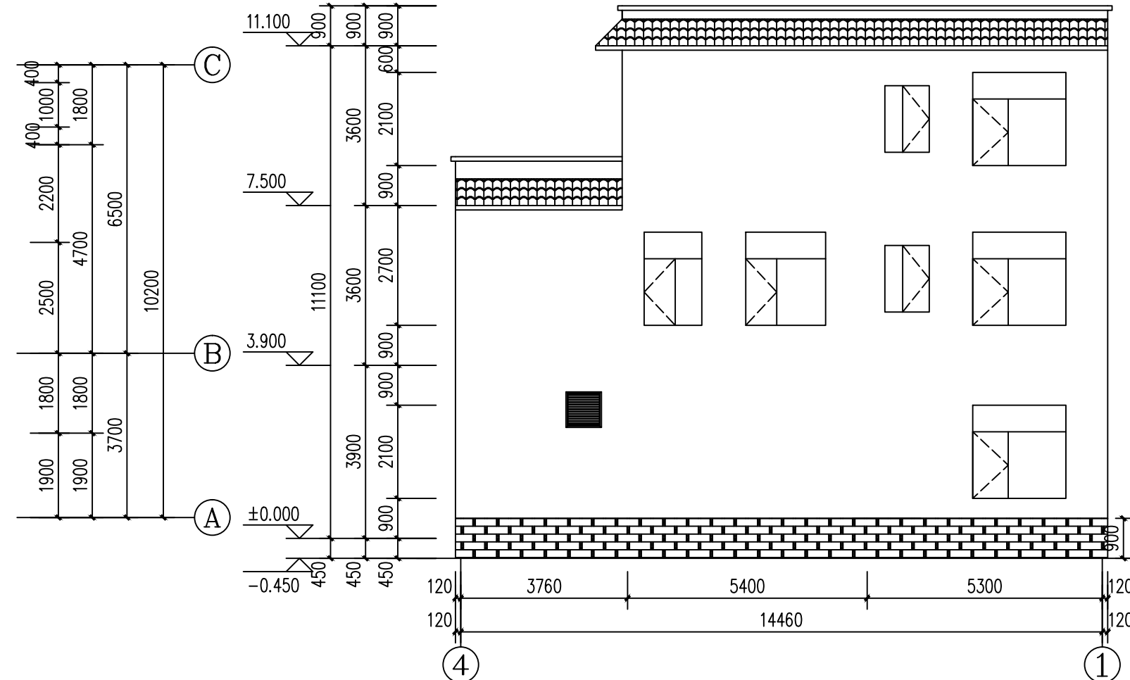
④-①立面图 1:100
