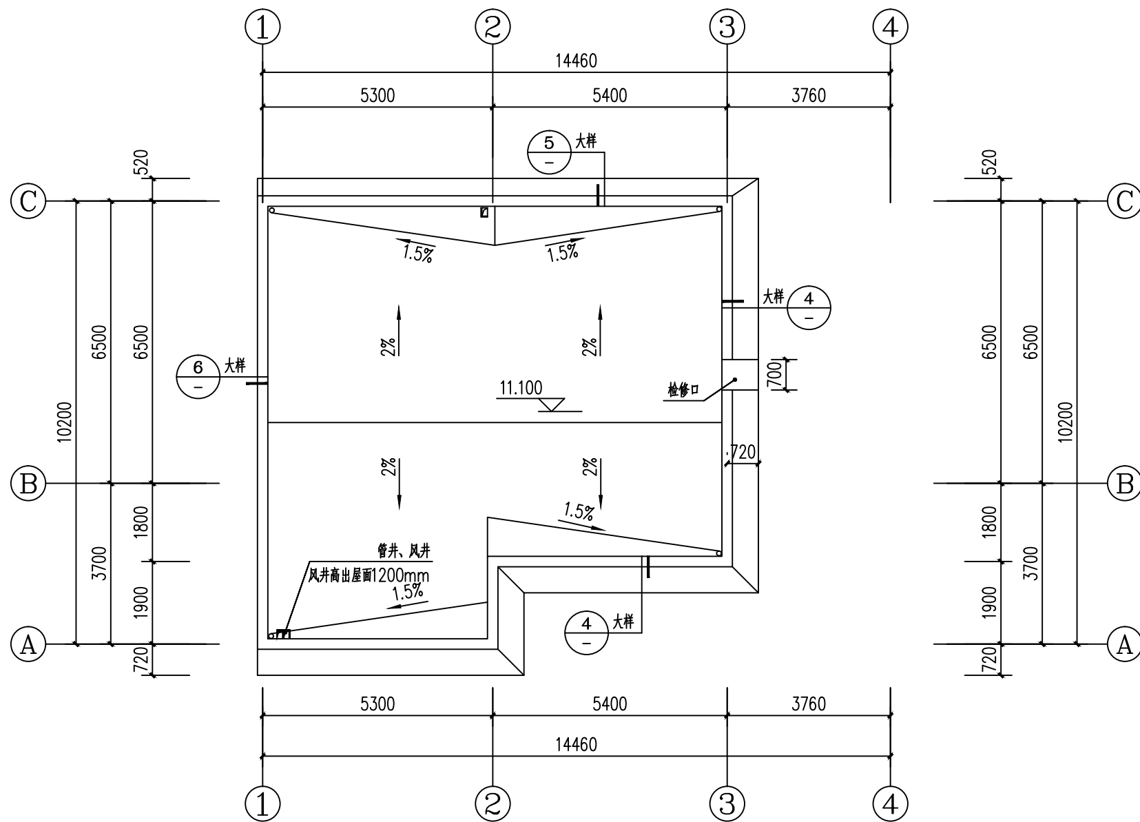
屋面平面图 1:100
