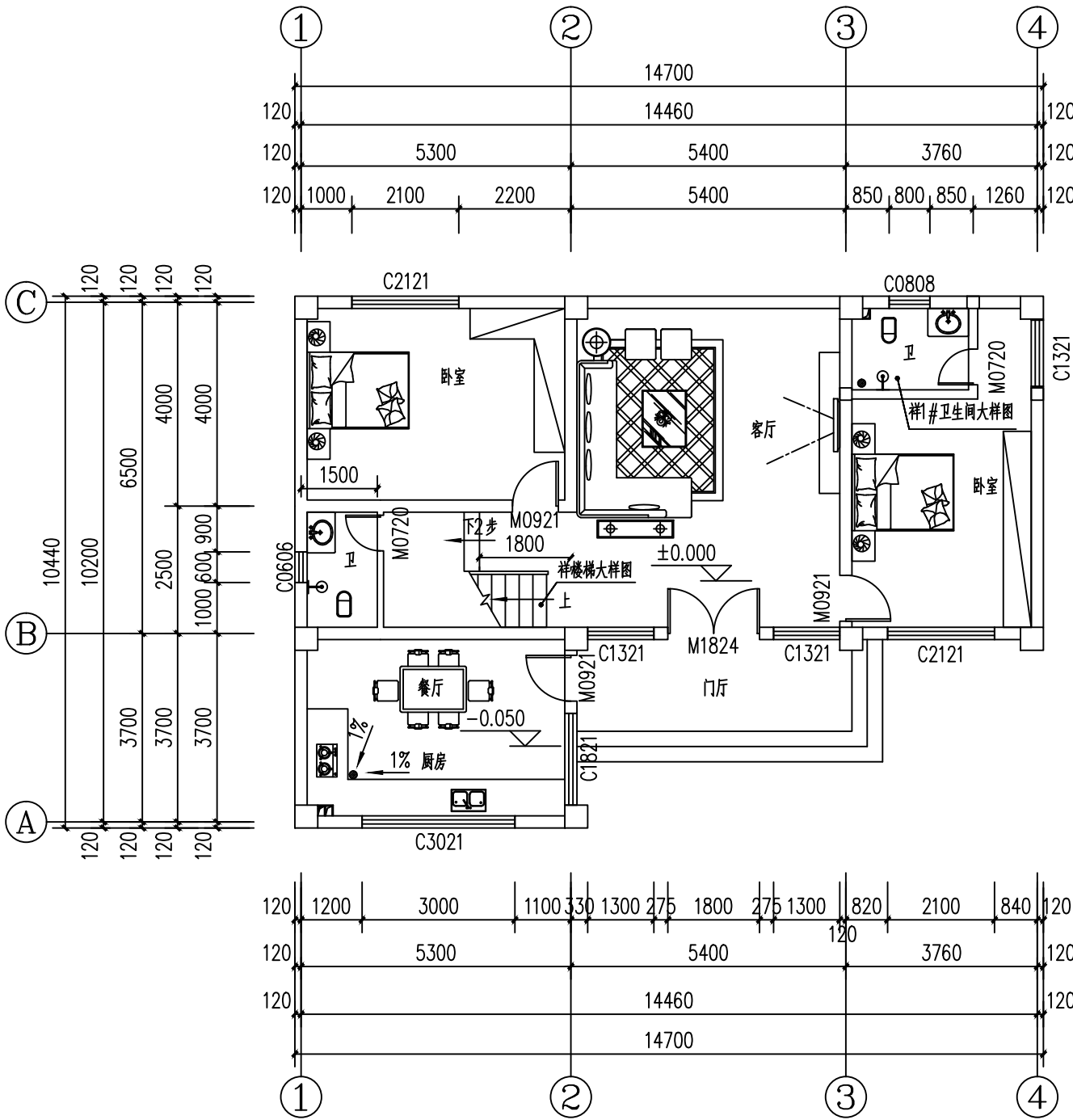
一层平面图 1:100
