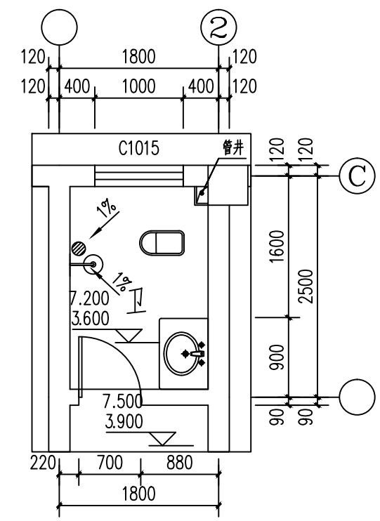
3#卫生间大样图 1:50
