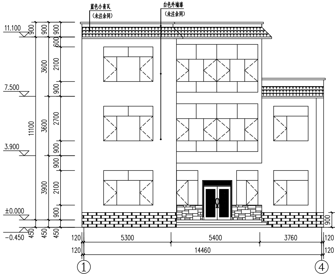
1-4立面图 1:100
