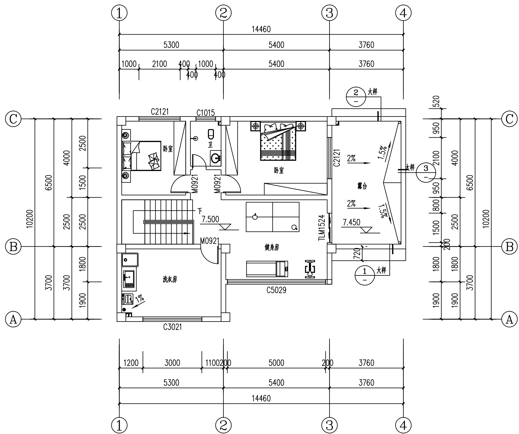
三层平面图 1:100
