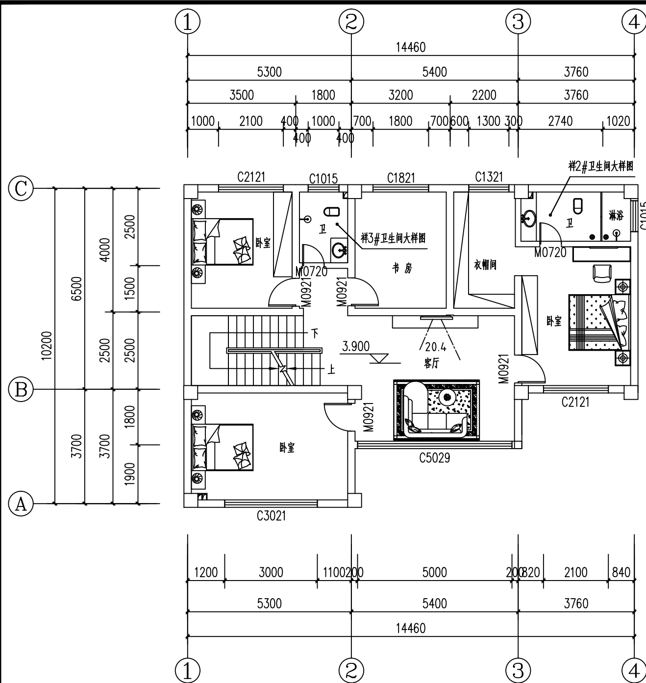
二层平面图 1:100
