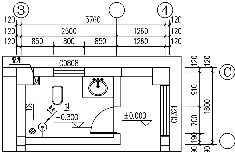
1#卫生间大样图 1:50
