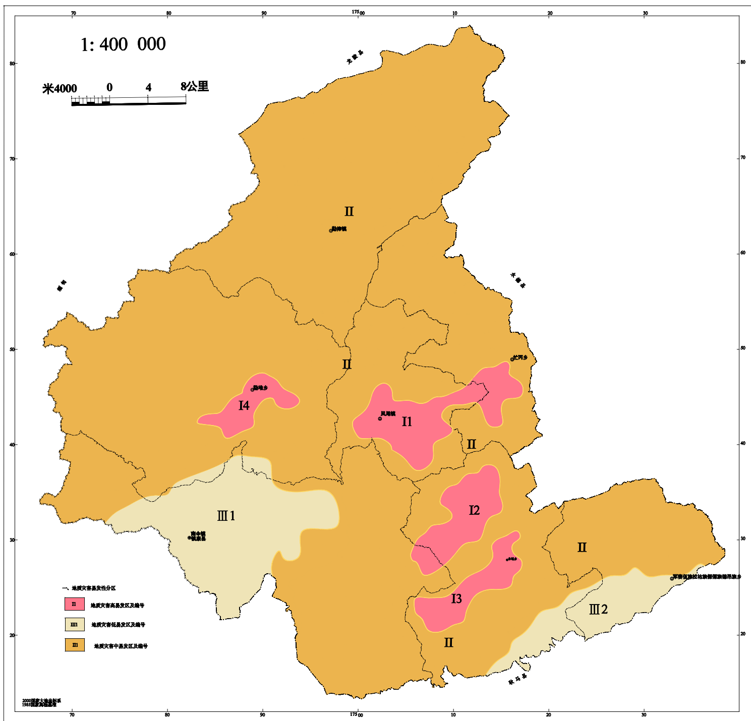
镇康县地质灾害易发性分区略图
